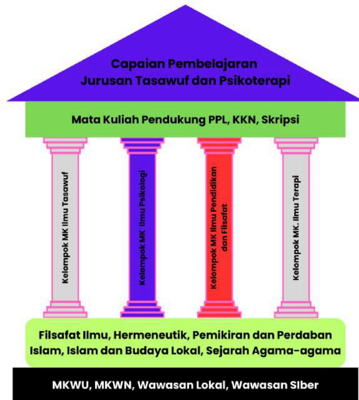
Gambar 1. Body of Knowledge Jurusan Tasawuf dan Psikoterapi
